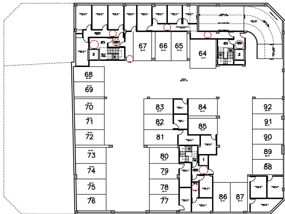
NIVEL -3
